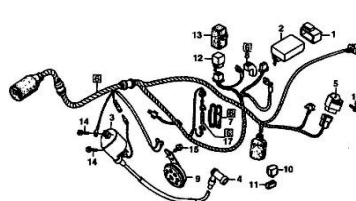
F27. WIRE HARNESS
