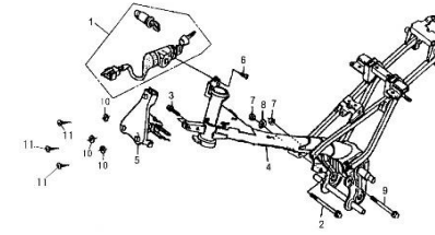
F28. FRAME BODY
